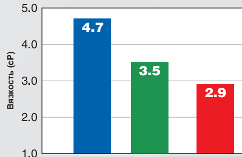
Сохранение вязкости при высоких температурах (ASTM D4683)
